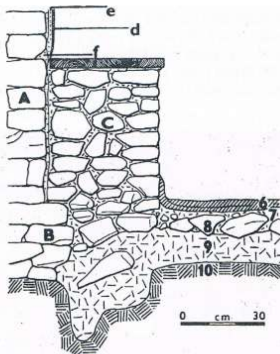
Obr. 19 Řez konstrukcí obvodové lavice v hlavní lodi Rotundy sv. Kateřiny ve Znojmě (B. Klíma 1995)
