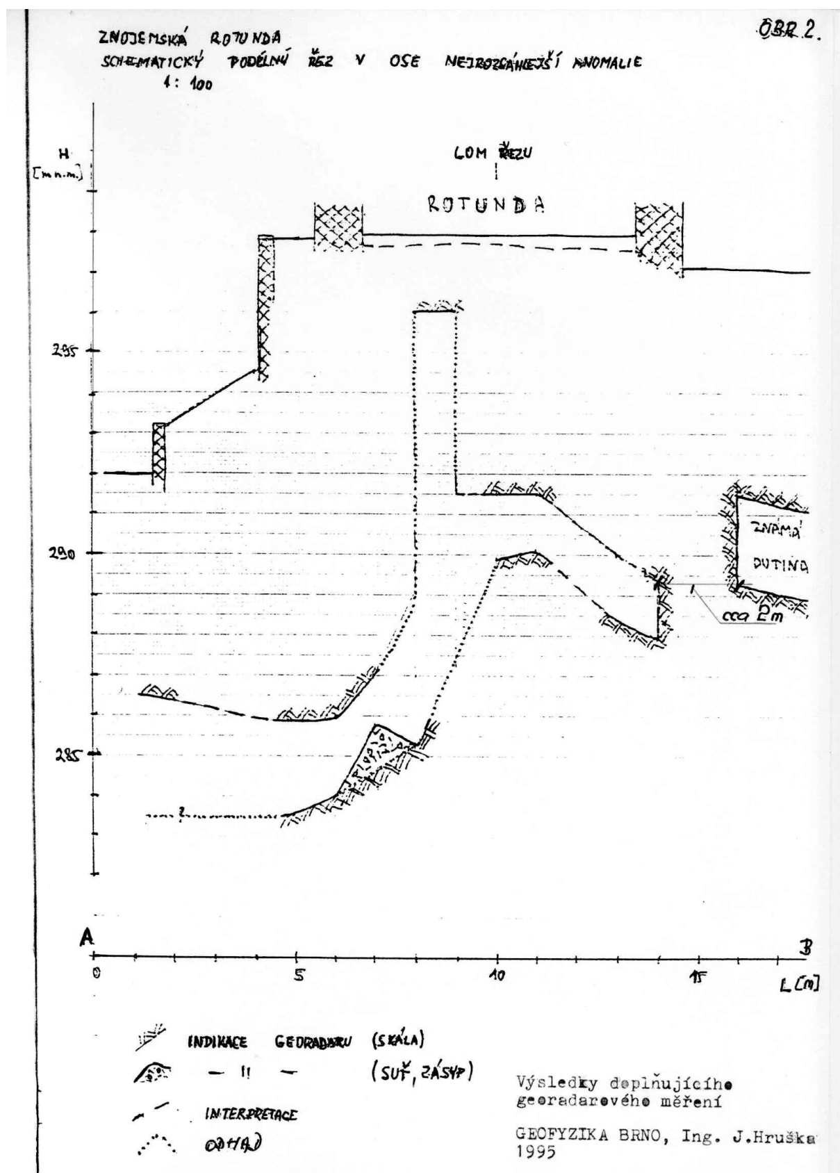
Příloha 8, (Obr. 2 Doplněk zprávy Geofyziky Brno o geofyzikálním měření –1995)
